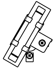
DETTAGLIO POSIZIONAMENTO DELLA RESISTENZA 470 SCALA 1/2
