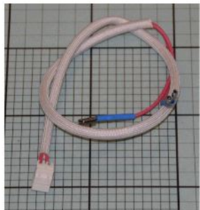
Cablage st16 : 36050713
